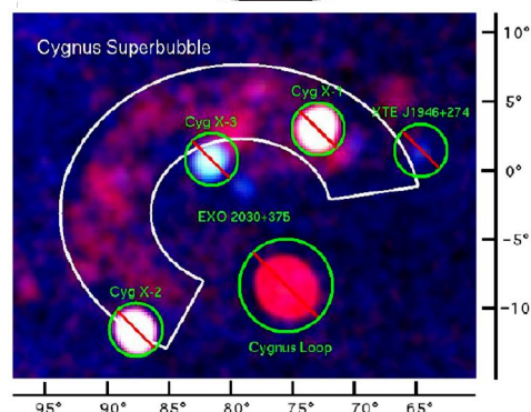
図: MAXI/SSC の X 線データによる全天図 (上) と Cygnus Super Bubble の拡大図 (下。白線の領域)。Kimura et al. 2012, arXiv:1211.3737 より引用。
